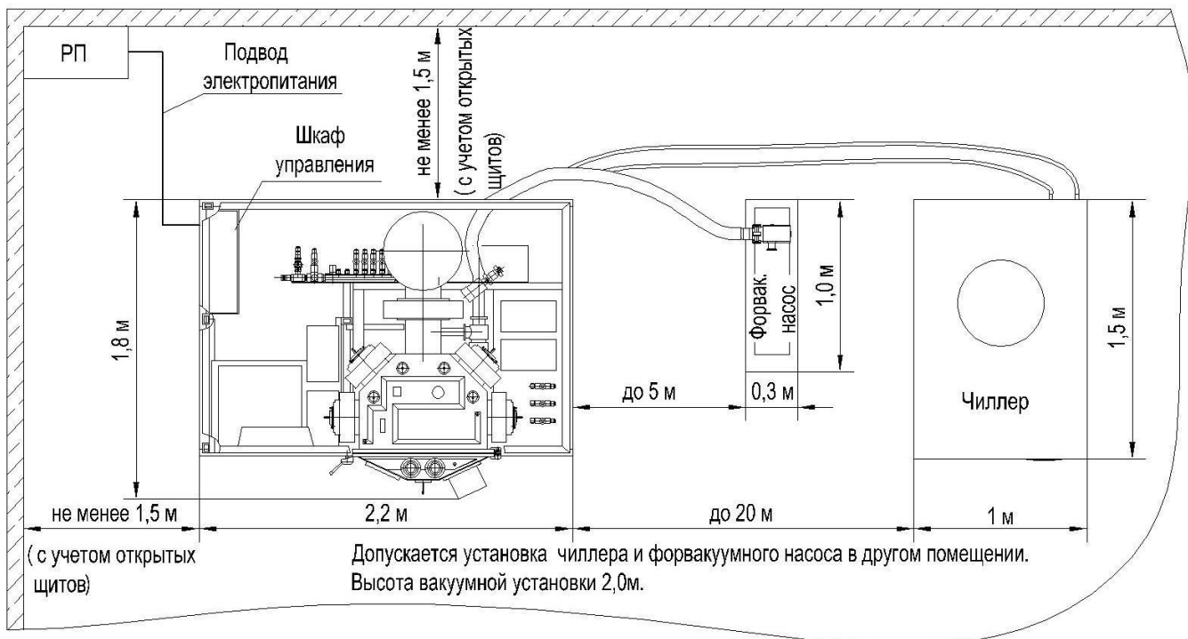
Примерное расположение вакуумной установки BRV 700-D
